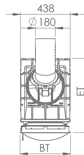
eurotherm 8/D Einbauversion
