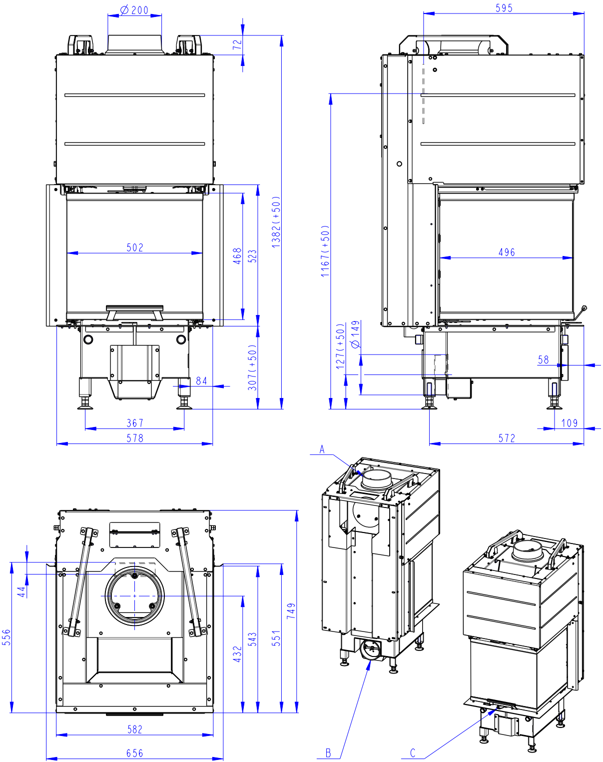
Dimension sketch, Maßzeichnung, Croquis des dimensions, Dimensioni ingombro
